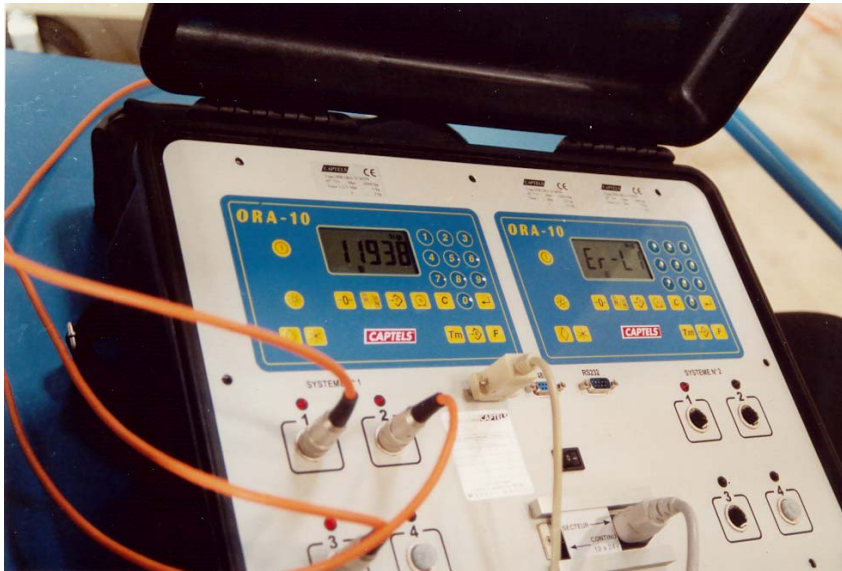
Equipo electrónico para determinación automática de centros de gravedad
